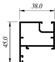
CIA-Co131 Nave
