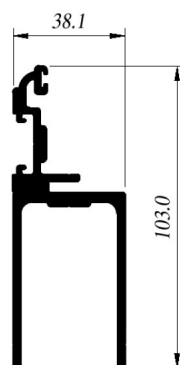
CIA-EI490 Zócalo Fijo
