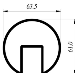
CIA-104063L Pasamanos
