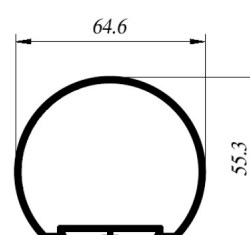
CIA-CH579 Pasamanos
