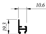
CIA-M114-M2 Inserto
