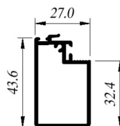
CIA-M158-M2 Enganche
