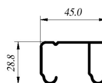
CIA-Co097 Riel
