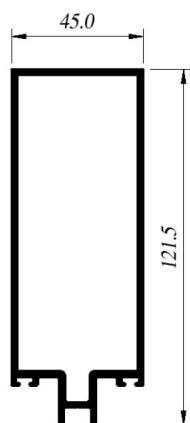
CIA-Co037 Vertical
