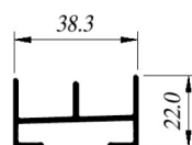
CIA-S201 Carrilera
