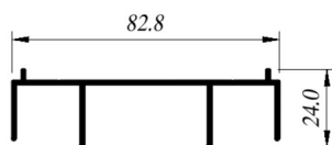
CIA-C151L Cabezal ALN-151
