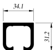
CIA-Co087 Riel Novo
