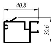
CIA-1672 Enganche
