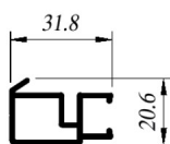
CIA-1642 Enganche
