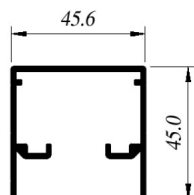
CIA-319 Cabezal
