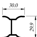
CIA-ALN827 Adaptador
