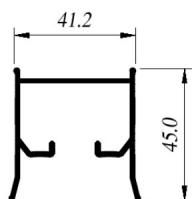
ALH-B-346-M Cabezal
