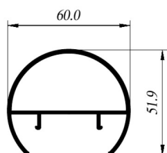
CIA-RD011 Pasamanos
