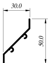
CIA-C315L8M Rejilla
