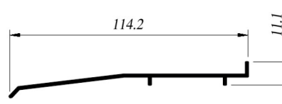
LS-36-1266 Alfajía
