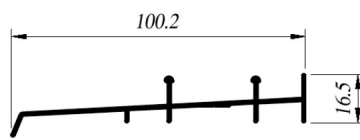
CIA-Co034 Sillar Alfajía ALN-386
