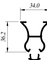
CIA-Co088 / 089 Refuerzo
