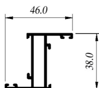
CIA-C176L Nave ALN-176
