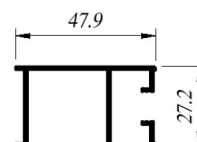
CIA-C190L Traslapo ALN-190L
