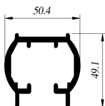
CIA-Co024 Cabezal
