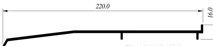
CIA-ALN449 Alfajía
