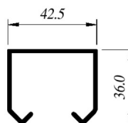
CIA-S391 Riel Closet
