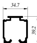
CIA-1764 Riel
