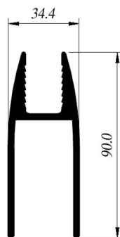
CIA-S369C Zócalo Móvil
