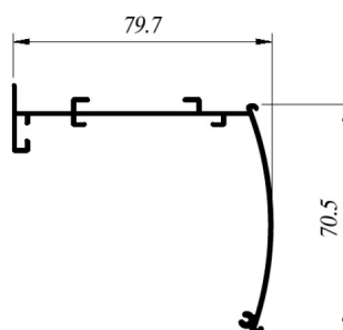
CIA-Co052 Cenefa
