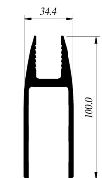
CIA-S351 Zócalo Fijo
