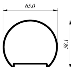
CIA-CoT144R Pasamanos
