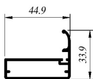
CIA-Co060 Marco
