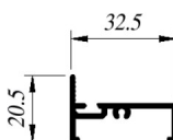
CIA-Co079 Marco C-Fijo
