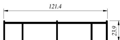
CIA-CR105 Cabezal 3 Rieles ALN-706
