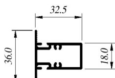
CIA-Co081 Divisor C-Fijo
