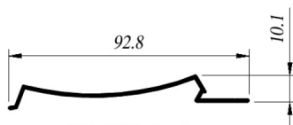
CIA-F007 Enchape
