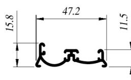
CIA-1768 Sillar
