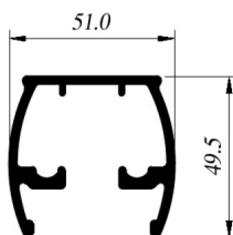
CIA-Co030 Cabezal
