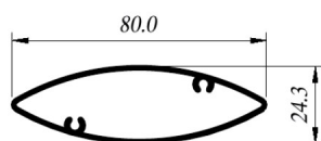
T-237 Quiebrasol
