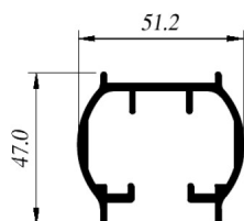
CIA-1769 Cabezal
