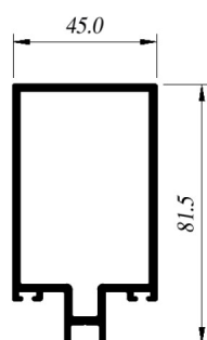
CIA-Co038 Horizontal
