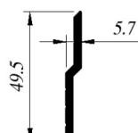
CIA-Co076 Soporte
