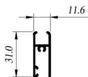
CIA-M122 Horiz. Inf.
