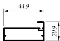
CIA-Co042M Marco
