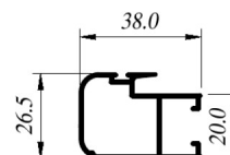
CIA-ALN1767 Enganche C.
