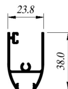
CIA-ALN874 Sup Curvo ALN-874
