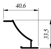
CIA-460 Soporte
