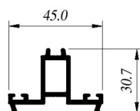
CIA-Co039M Adaptador V-Doble
