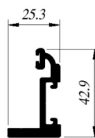
CIA-EI491 Compl. Zócalo
