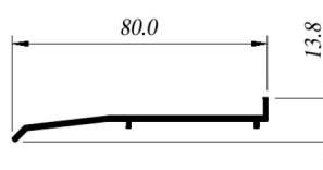
ALN-1122 Alfajía
