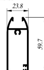
CIA-ALN875 Inf Curvo ALN-875
