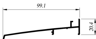
CIA-1551 Sillar Alfajía
