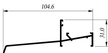
CIA-Co093 Sillar Alfajía
