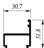
CIA-Co094 Inserto
