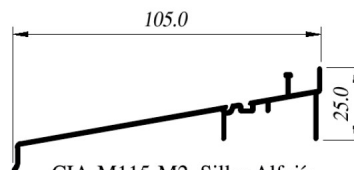
CIA-M115-M2 Sillar Alfajía
