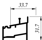
CIA-M160 Sillar Camara
