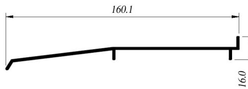
ALN-413 Alfajía
