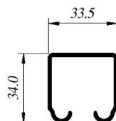
CIA-Co096C Riel
